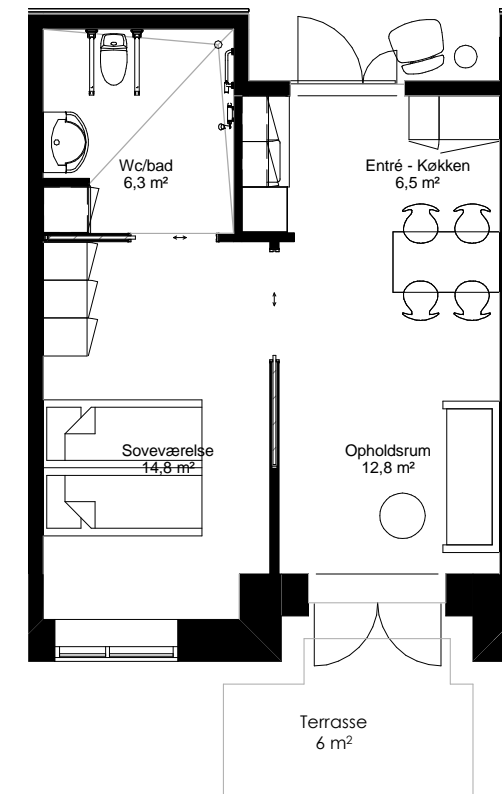
Indretningsplan Copy 1 Copy 1 1 : 100
