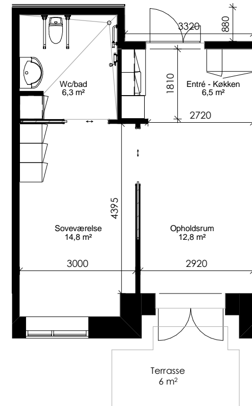
Indretningsplan Copy 1 1 : 100
